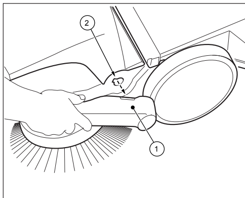
Bild 14: Nedmontering av skjutbygel (haaga 477 / 497 Profi)
