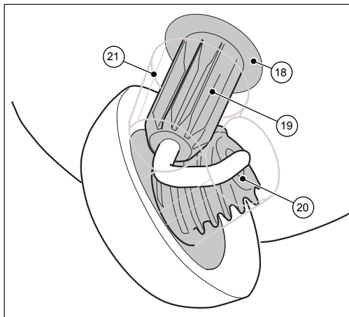
Abb. 4: Komponentenansicht 4
