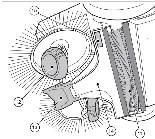
Kuva 2: Laitteen osat 2
