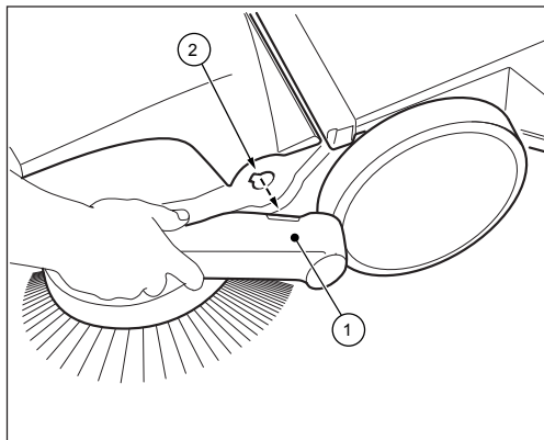
Kuva 14: Työntöaisan irrottaminen (haaga 477 / 497 Profi)
