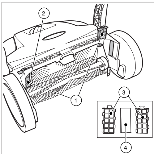
Kuva 12: Pölynsuodattimen poistaminen
