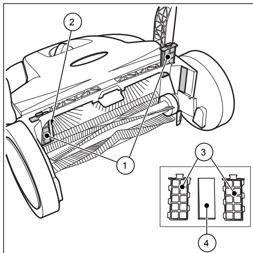
Рис. 12: Извлечение пылесадерживающих фильтров
