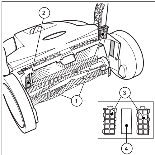
Abb. 12: Staubfilterentnahme
