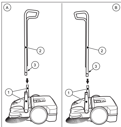
Bild 8: Montera skjutbygeln
