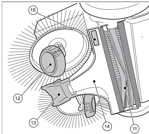
Fig. 2: Komponentoversikt 2
