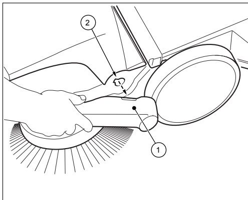
Rys. 14: Demontaż uchwytu do przesuwania (haaga 477 / 497 Profi)
