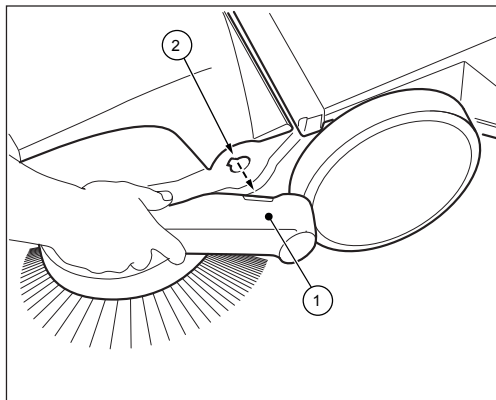
Fig. 14: Desmontaje del manillar (haaga 477 / 497 Profi)
