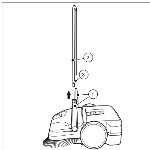
Bild 13: Nedmontering av skjutbygel (haaga 375)
