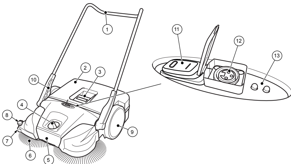
Fig. 1: Komponentoversigt 1
