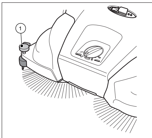
Abb. 14: Niederhaltereinstellung
