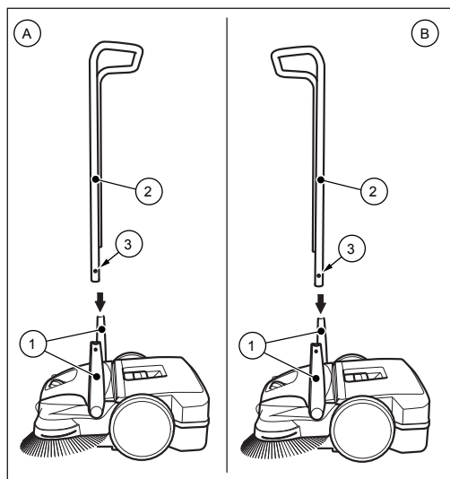
Abb. 8: Schiebebügelmontage
