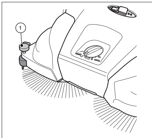
Fig. 14: Nedholder indstilling
